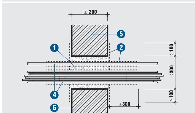
Detal A - Widok przejścia kablowego
