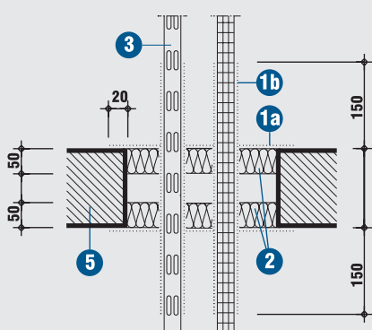
Detal B - Przeście kablów przez strop
