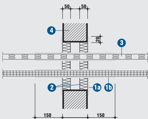
Detal A - Przeście kablów przez ścianę
