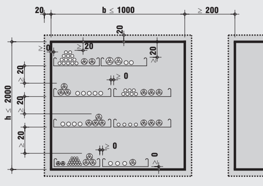
Detal C - Widok przeście kablów
