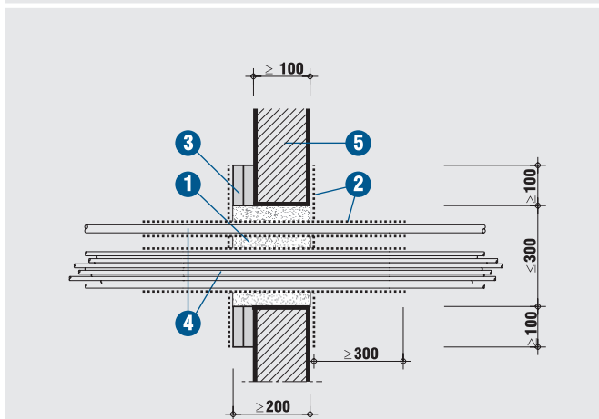
Detal B - Zwiększenie grubości ściany
