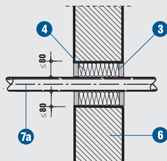
Detal A - Przejście rur stalowych i żeliwnych o średnicach nie większych niż 40mm przez ścianę i strop
