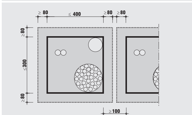
Detal A - Widok przejścia kablowego
